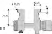
ab 25 mm
